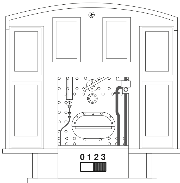
Bild 1, Betriebsartenschalter
