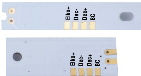
Abbildung 2: Anschlussmöglichkeiten und Pufferanschluss Figure 2: Advanced hook up with power buffer
